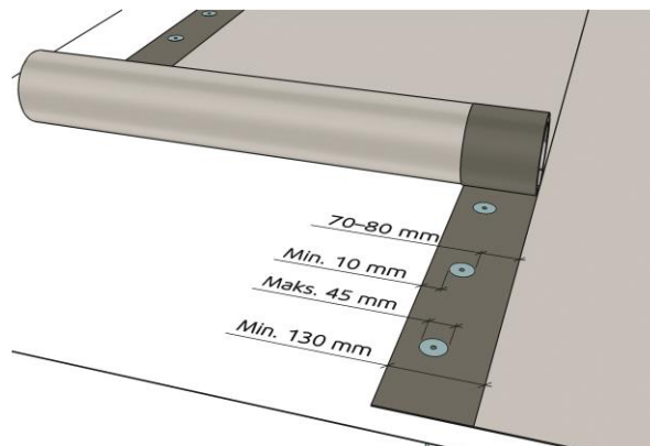
Fig. 1 EshaFlex TOP Mono ettlags asfalt takbelegg festes mekanisk i omlegget som sveises.
